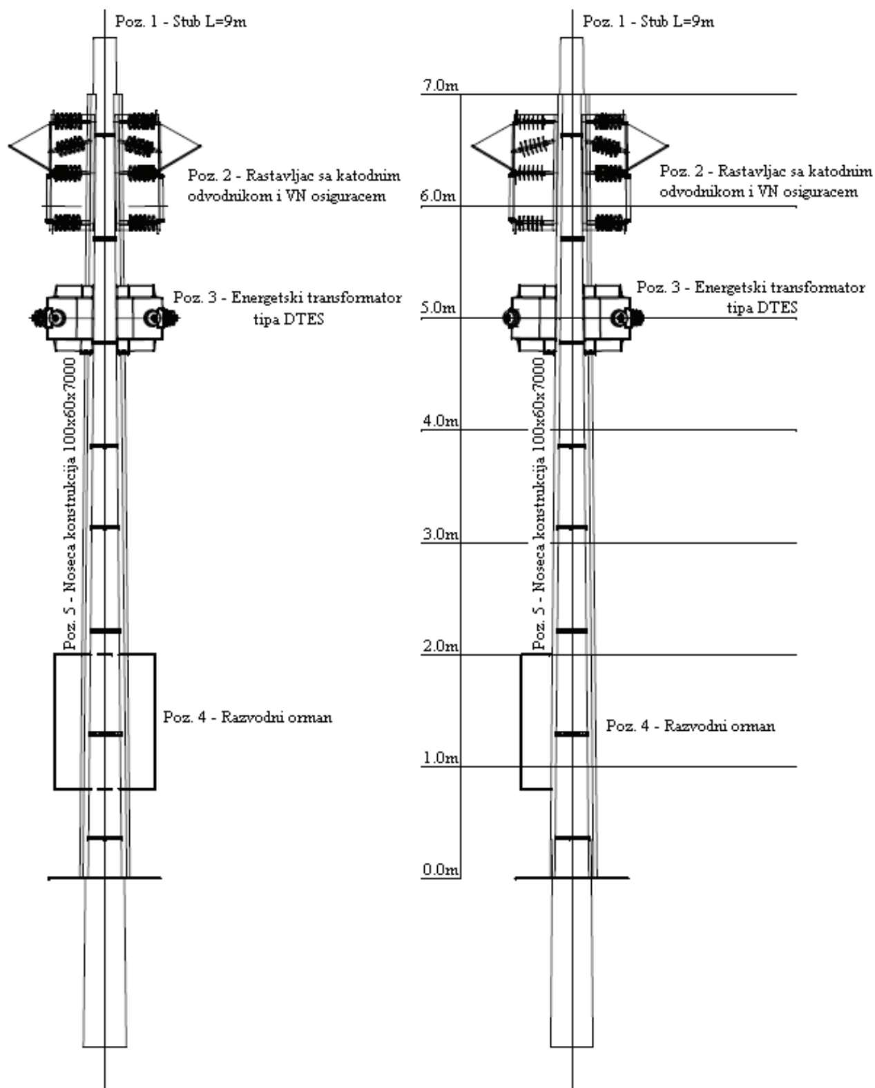
Izgled STS 10/0.42 kV/kV sa merenjem na niskom naponu
