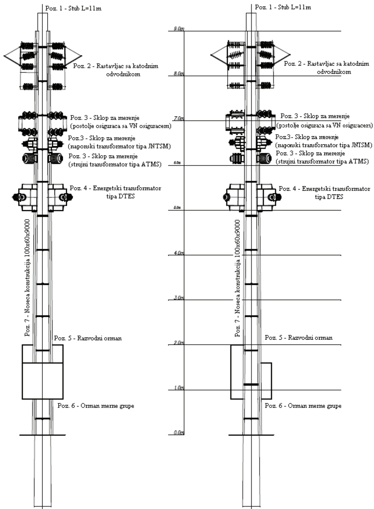
Izgled STS 10/0.42 kV/kV sa merenjem na srednjem naponu
