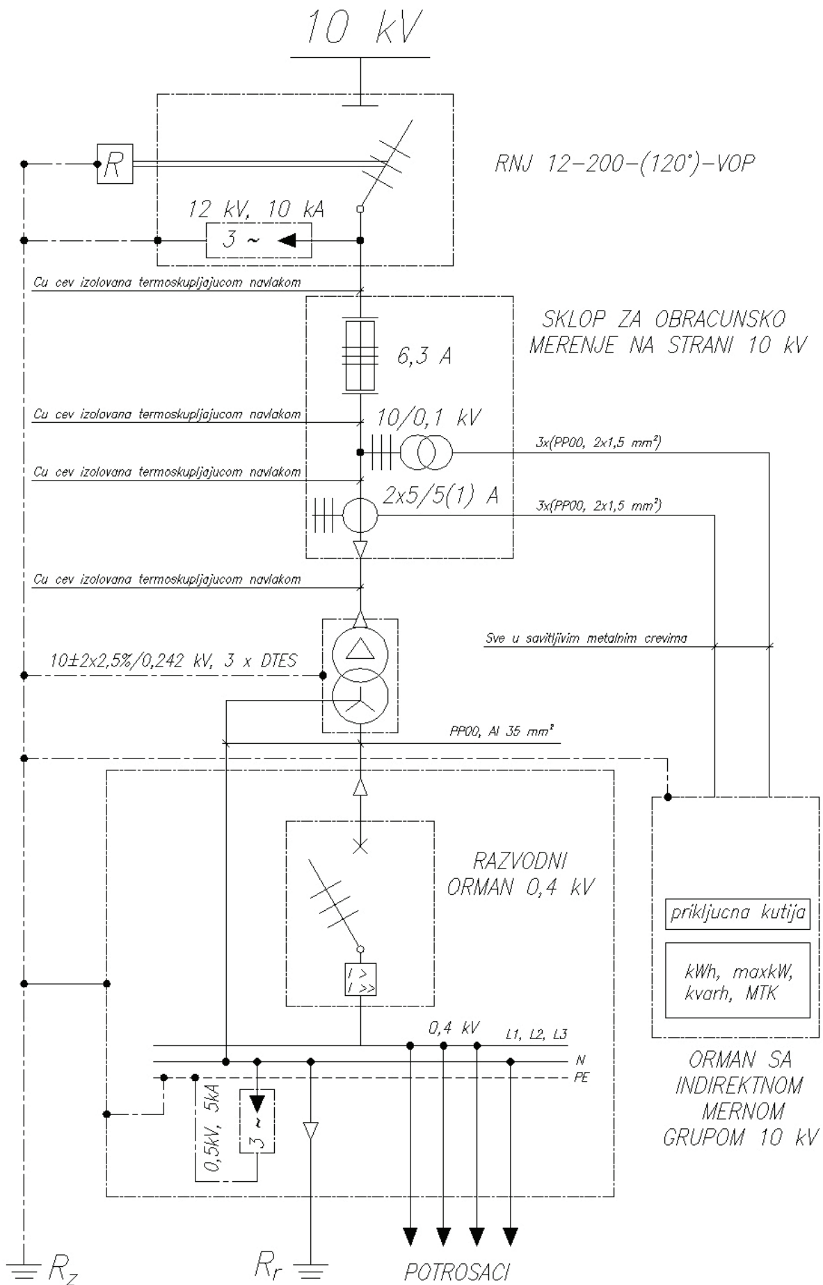
Jednopolna šema STS 10/0.42 kV/kV sa merenjem na srednjem naponu
