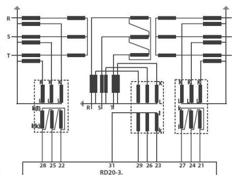
Diferencijalna zaštita transformatora Yy0d5 (oznake u zagradi važe za spregu Yy6d5)
