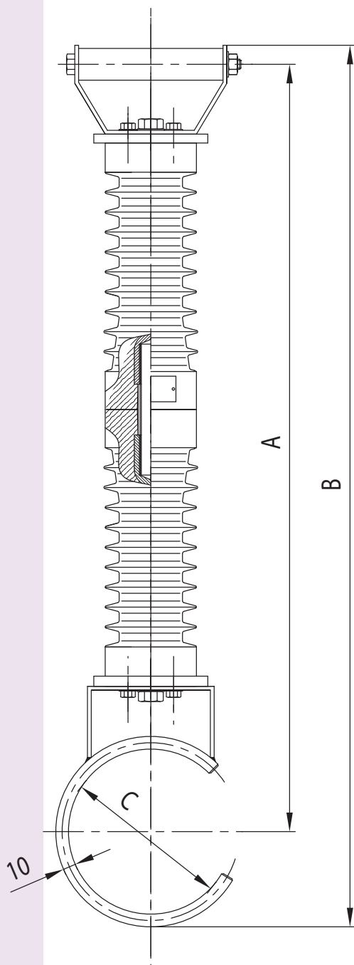
NOSAČ VN KABLA NVK
