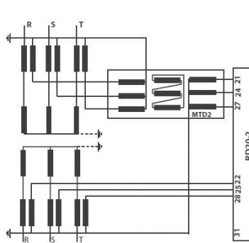
Diferencijalna zaštita transformatora Yy
