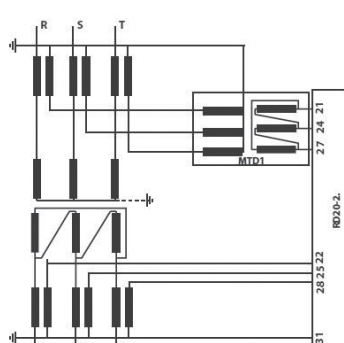
Diferencijalna zaštita transformatora Yd
